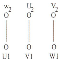
ÜÇGEN BAĞLANTI
