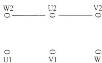
YILDIZ BAĞLANTI
