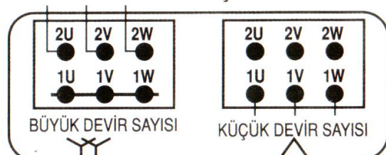
ÇİFT DEVİRLİ (DAHLENDER) MOTOR BAĞLANTI ŞEMASI
